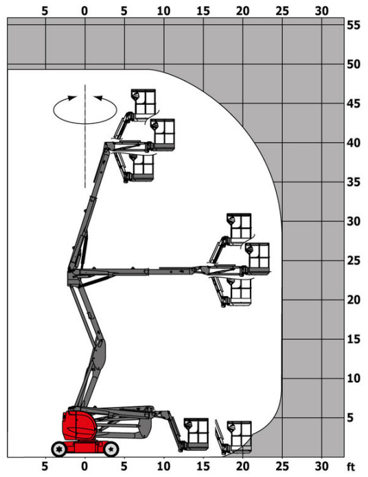
Abaque de charge impériale
